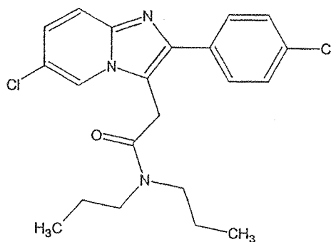
Alpidem
