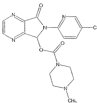
Zopeclon
