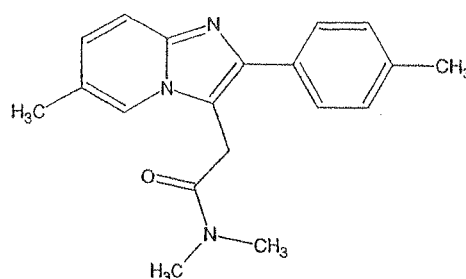
Zolpidem
