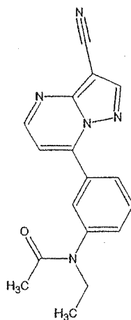
Zaleplon
