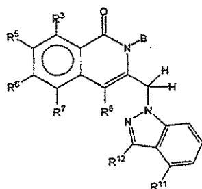
Formula VI-A
