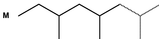
isobutyl end group
