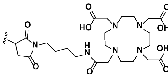
maleimide-nBu-DOTA
