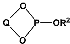
Structure VIIb
