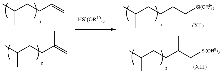
Scheme VI
