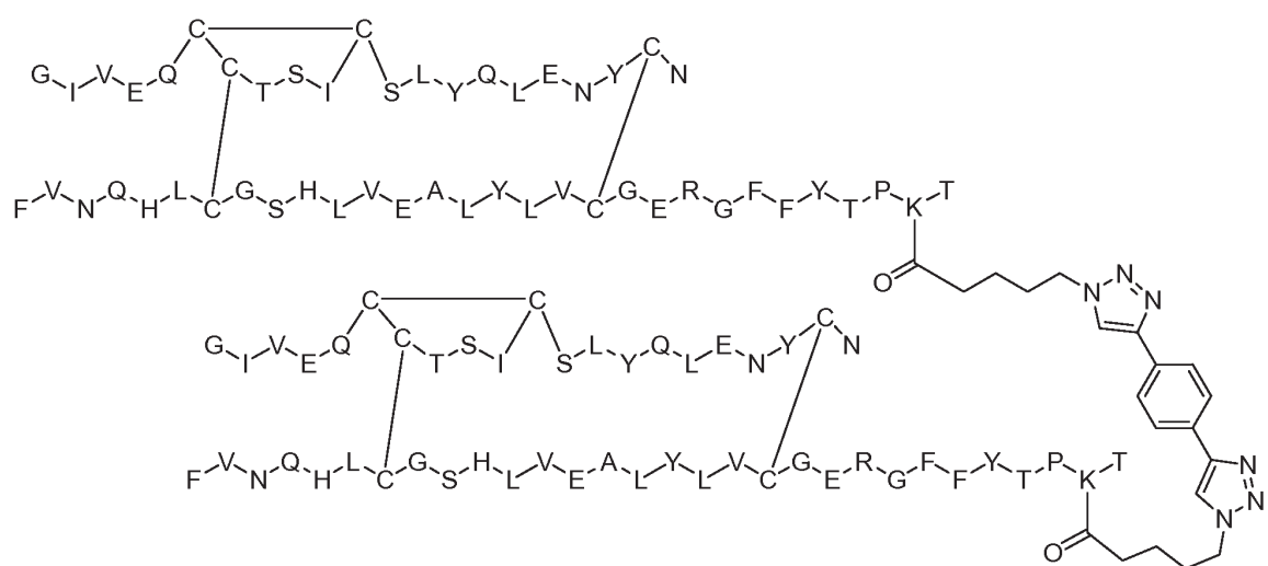
Dimer 59;
