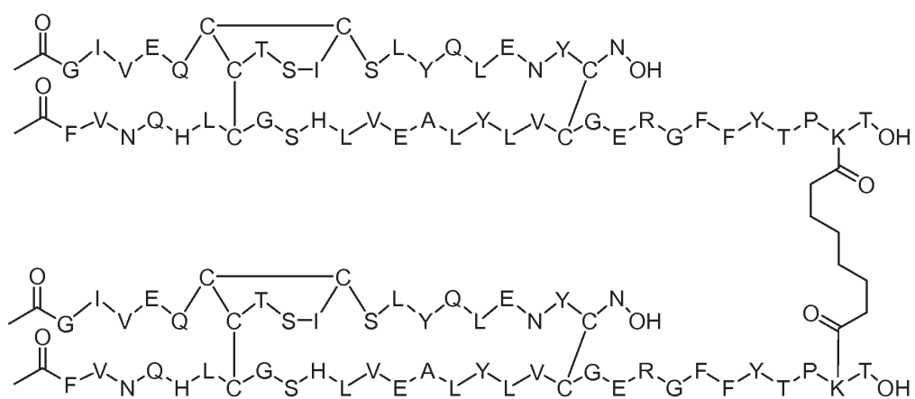
Dimer 55;
