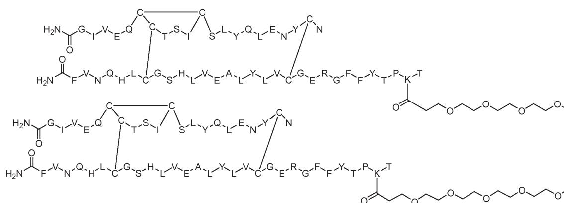
Dimer 15;
