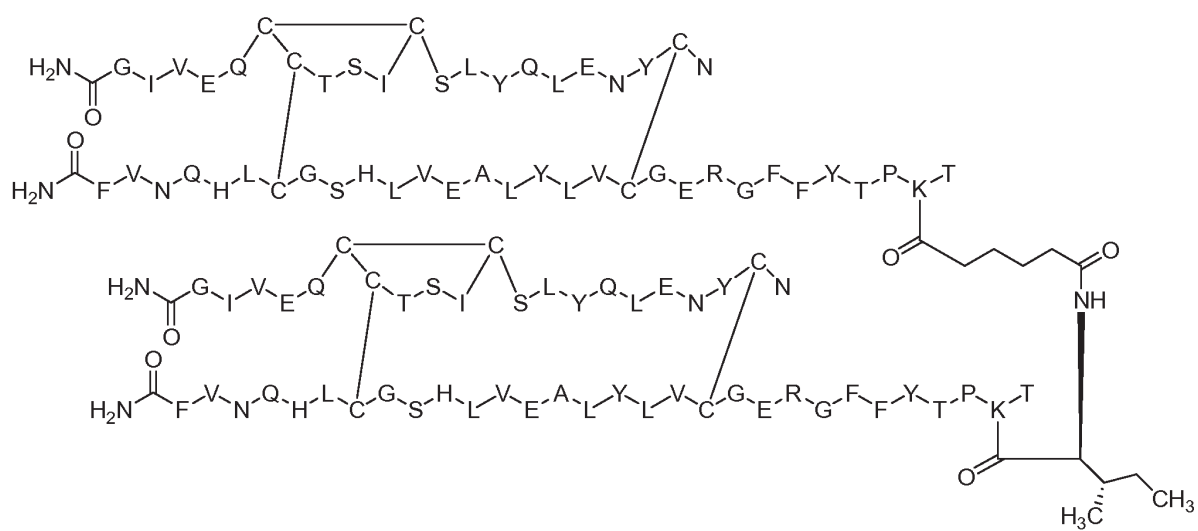
Dimer 63;
