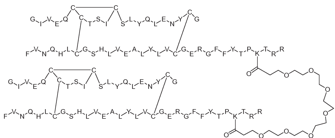
Dimer 53;
