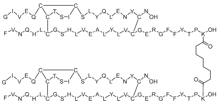
Dimer 20;
