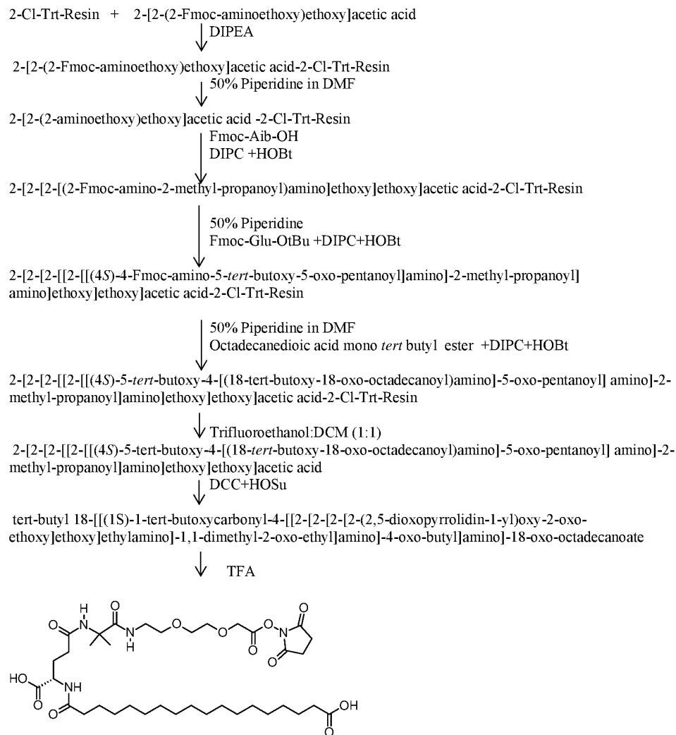
Moiety D-OSu
