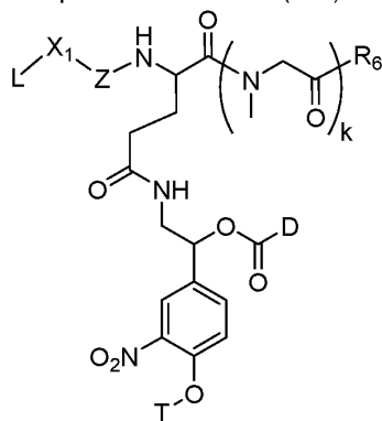
(VIII)
