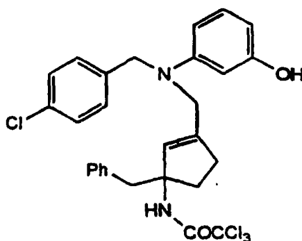
Cpd. 28
