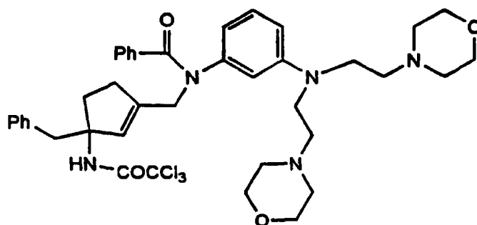
Cpd. 23b
