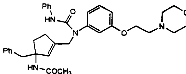
Cpd. 15
