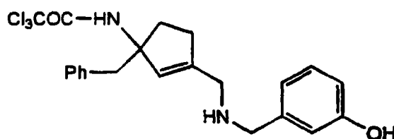
Cpd. 30
