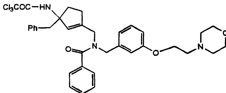
Cpd. 32
