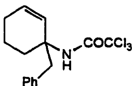
Cpd. 3
