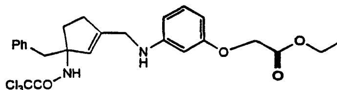
Cpd. 43
