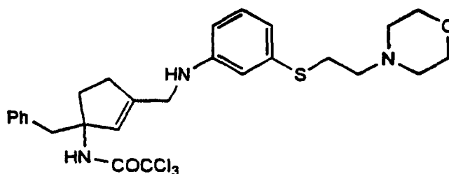
Cpd. 21
