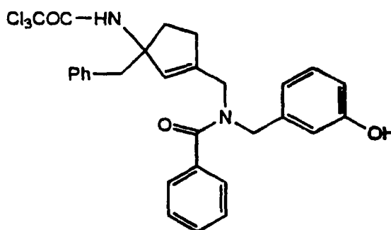
Cpd. 31
