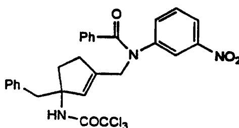
Cpd. 24
