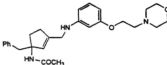
Cpd. 14
