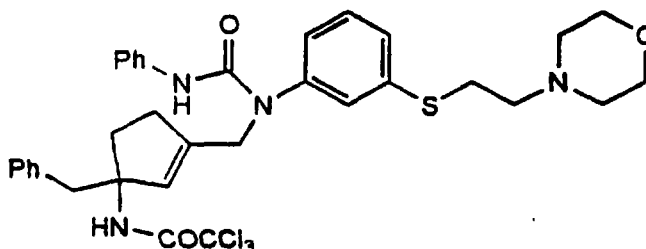
Cpd. 22
