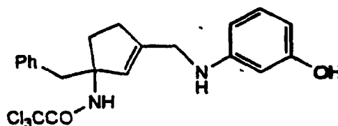
Cpd. 42
