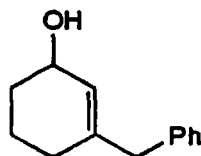
Cpd. 2
