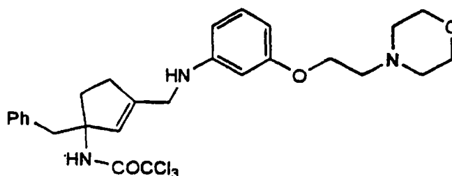
Cpd. 6
