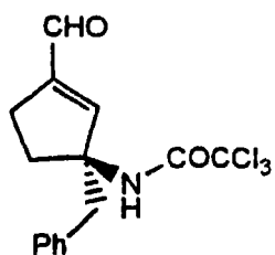
Cpd. 4a
