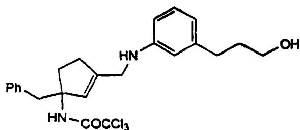
Cpd. 17
