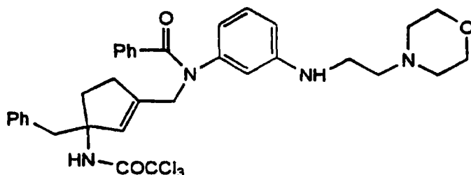
Cpd. 23a
