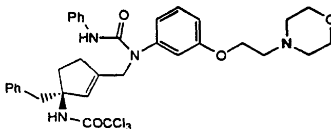
Cpd. 9
