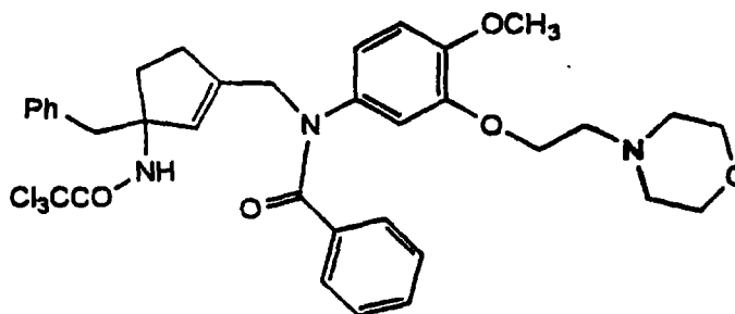
Cpd. 41
