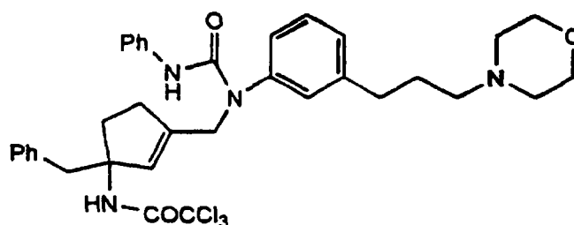
Cpd. 19
