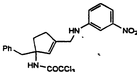
Cpd. 23
