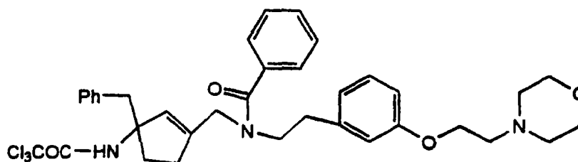
Cpd. 34
