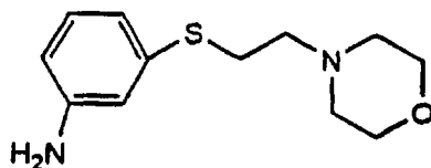
Cpd. 20
