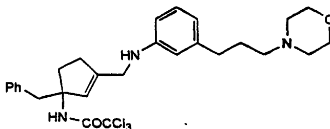
Cpd. 18
