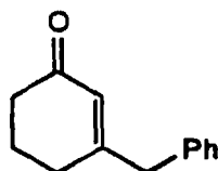
Cpd. 1
