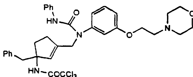
Cpd. 7
