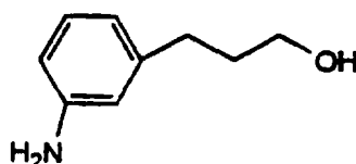
Cpd. 16
