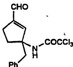
Cpd. 4
