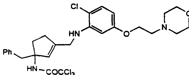
Cpd. 37
