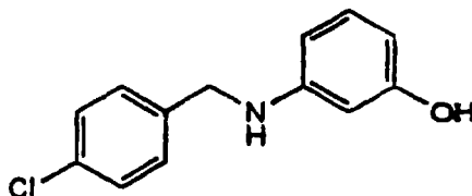
Cpd. 27
