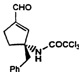
Cpd. 4b
