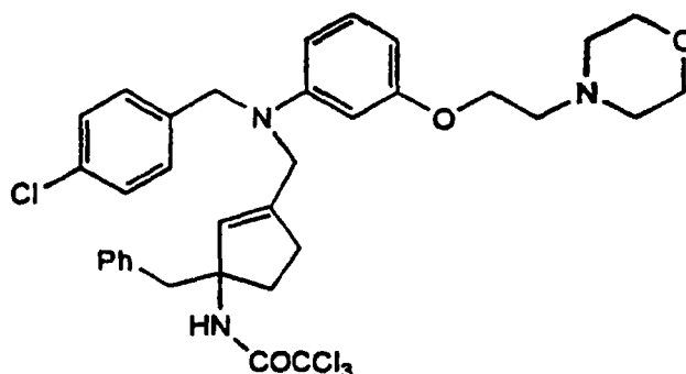
Cpd. 29
