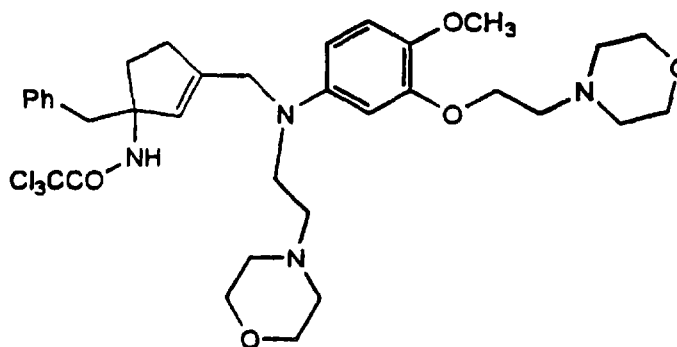
Cpd. 40
