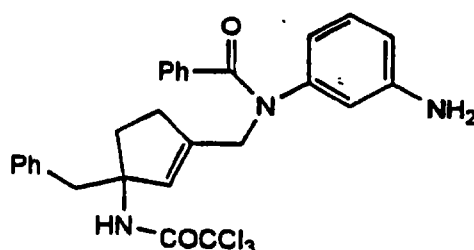
Cpd. 25
