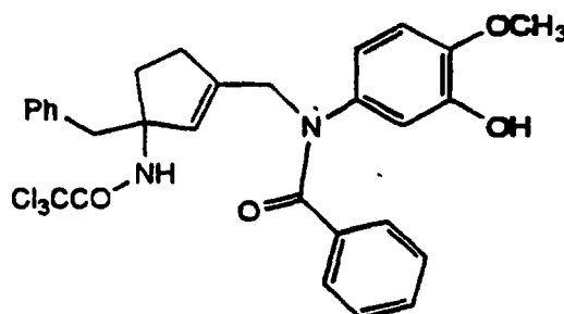
Cpd. 41
