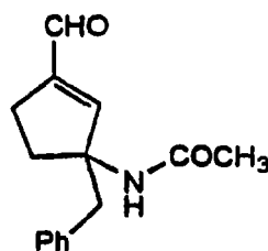
Cpd. 13
