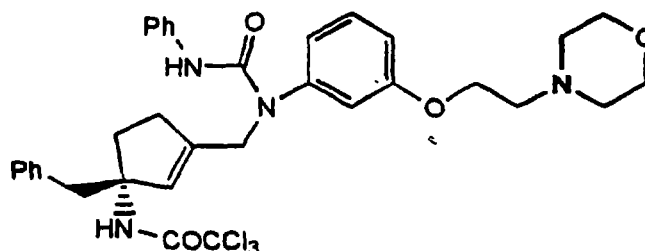
Cpd. 8
