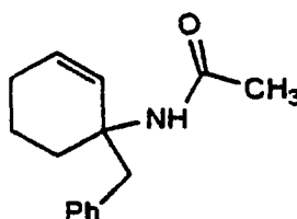
Cpd. 12
