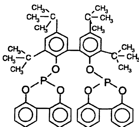
Ligand F
