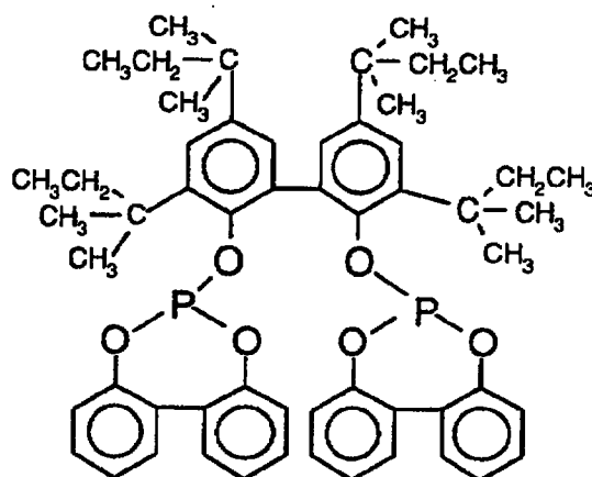
Ligand E
