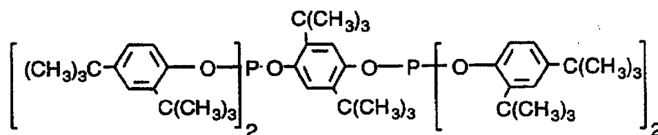
Ligand T
