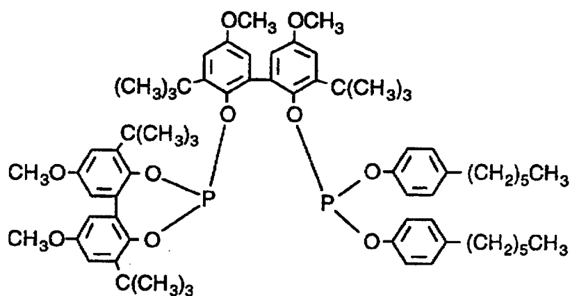
Ligand Q
