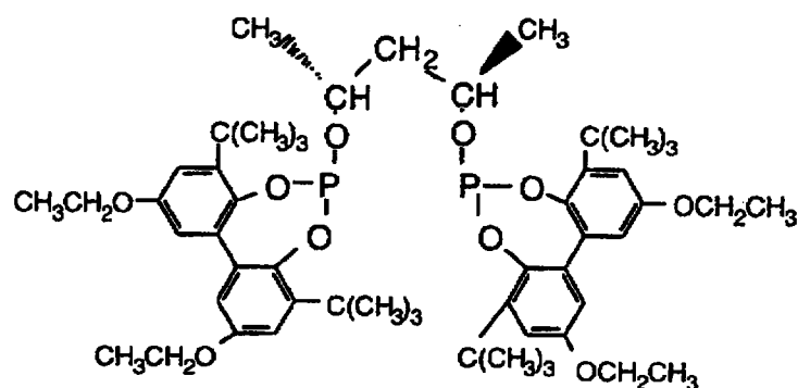
Ligand K
