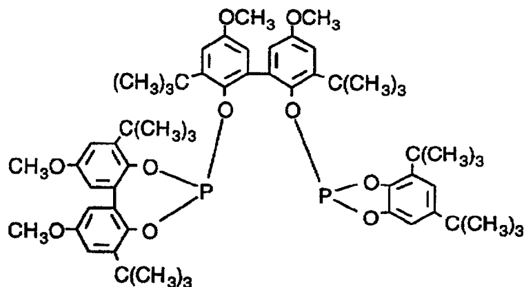
Ligand N
