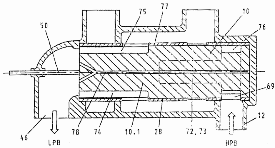
Fig. 9 (A - A)
