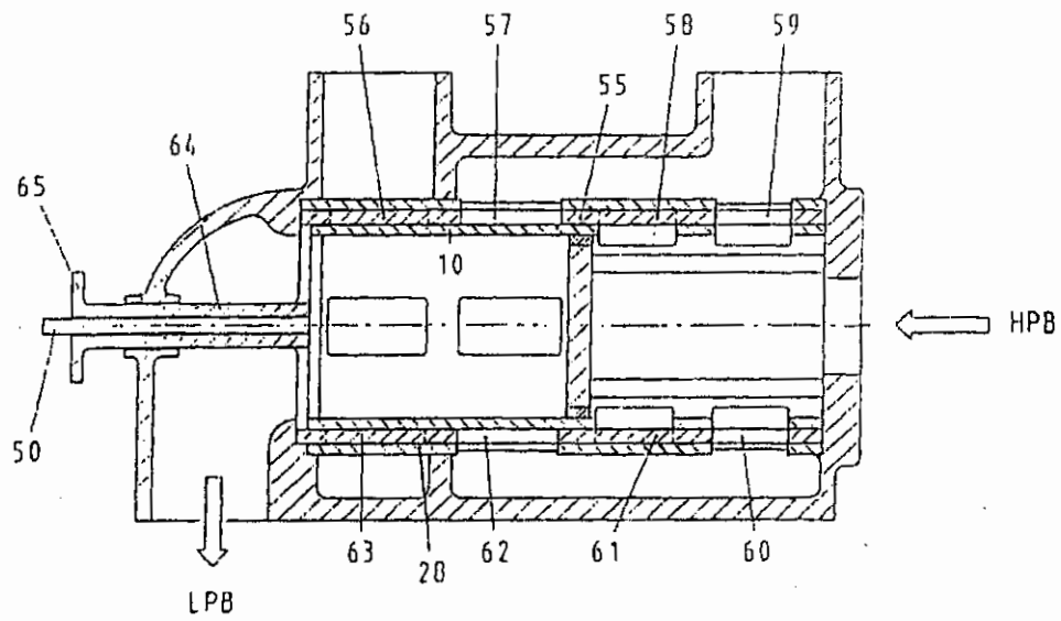
Fig. 7 (A - A)
