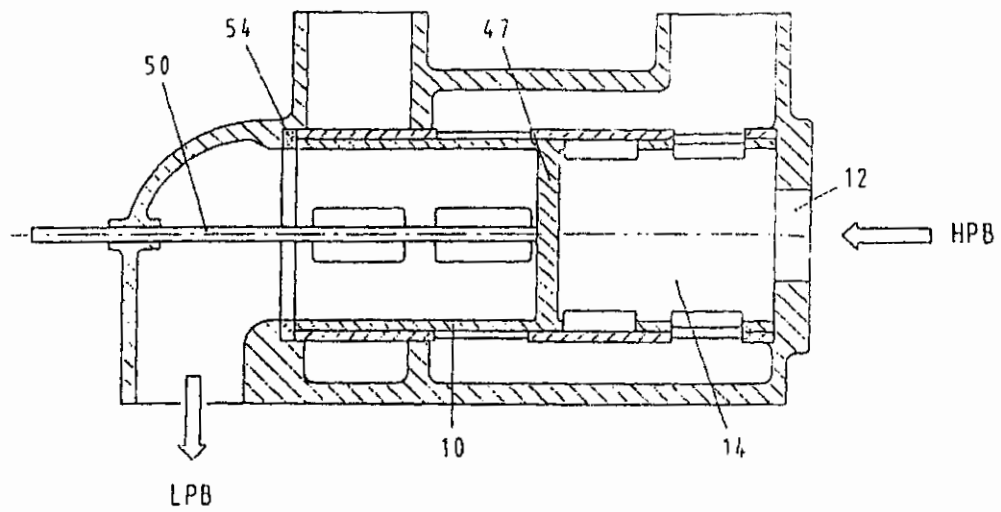
Fig. 6 (A - A)
