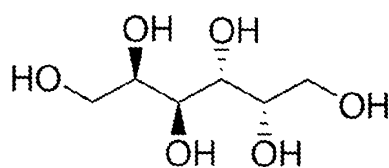
Dulcitol.
