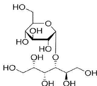
Maltitol, or
