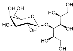
Lactitol.
