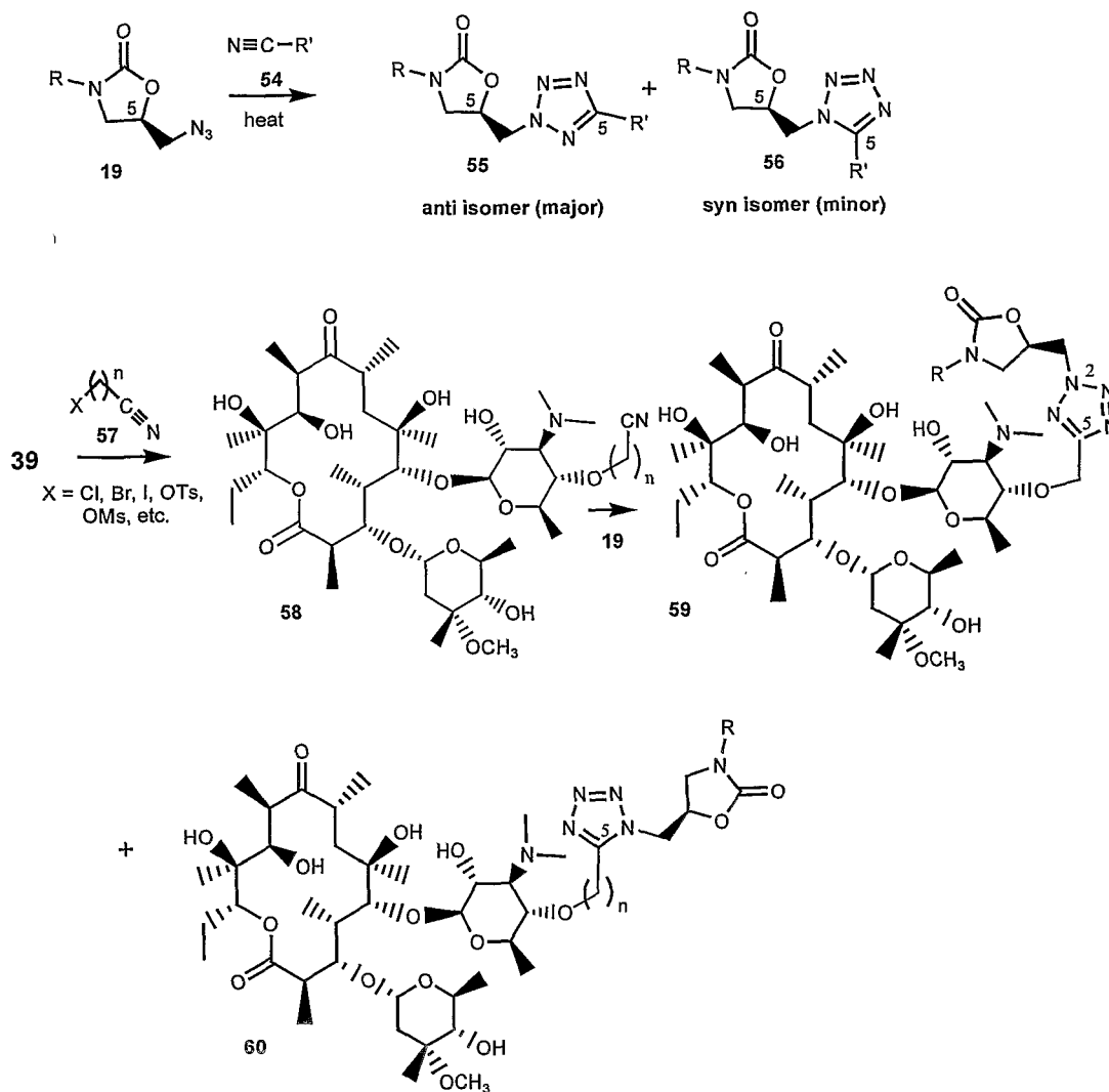
Scheme 8a
