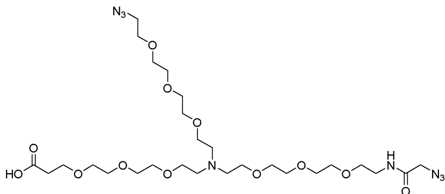
N-(PEG 3 -acid)-N-(PEG 3 -azide)-N-(PEG 3 -NH-AcAz);
