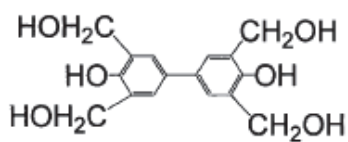
TML-BP
