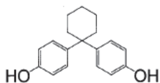
Bis-Z
