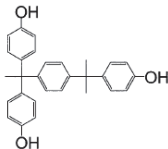
TrisP-PA
