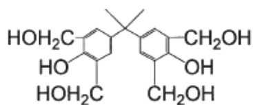
TM-BIP-A
