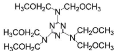
NIKALAC MW-100LM
