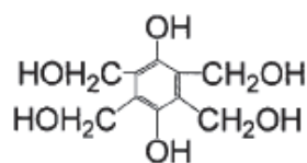
TML-HQ
