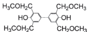
TMOM-BP
