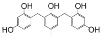
BIR-PC
