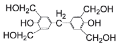
TML-pp-BPF
