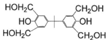
TML-BPA
