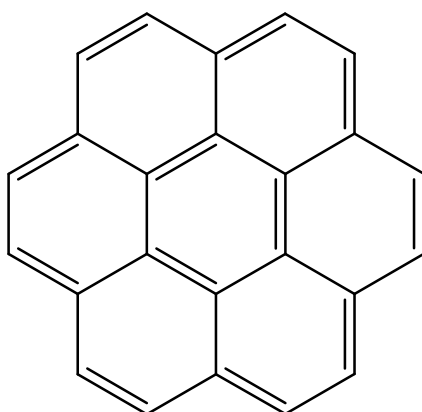
coronene
