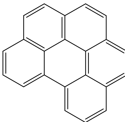
benzo(ghi)perylene
