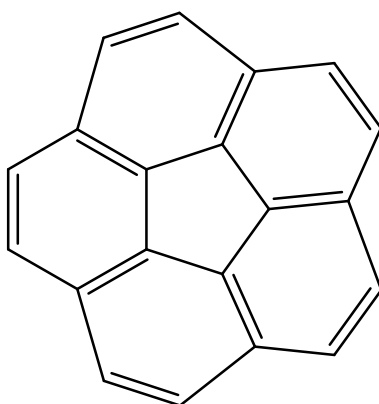
corannulene
