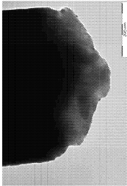
Ni/ZrO 2
