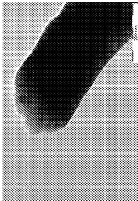
ZnO/ZrO 2
