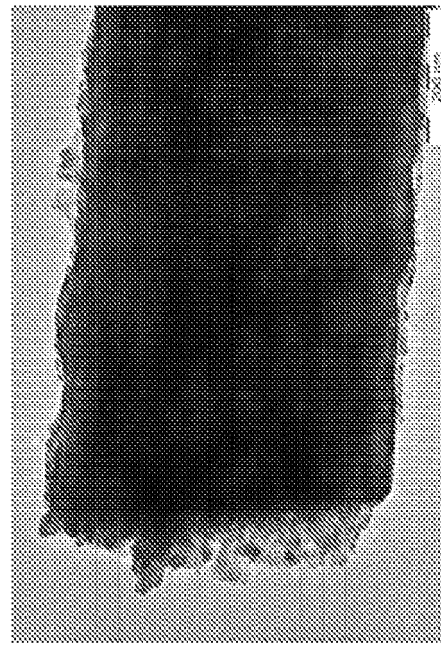
Fe/ZrO 2
