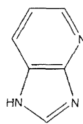
4-Azabenzimidazole
