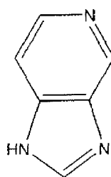
5-Azabenzimidazole
