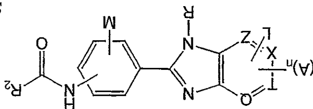
Supragenus A;
