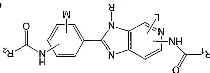
Genus D2
