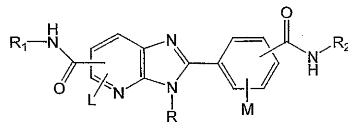
Genus A5
