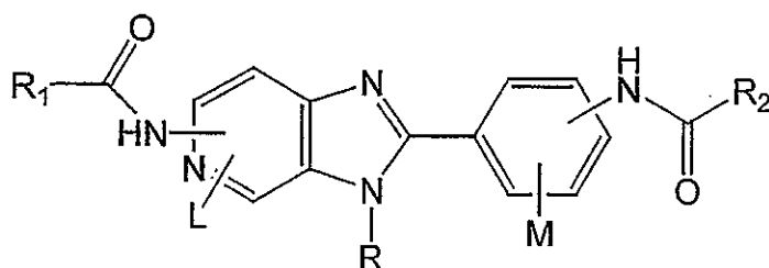
Genus D2;
