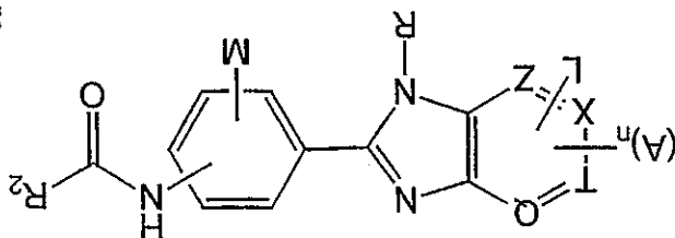
Supragenus A;
