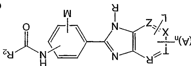
Genus A5
