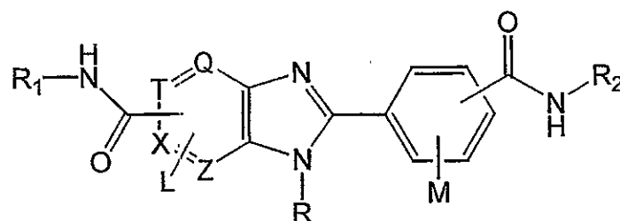
Supragenus B;
