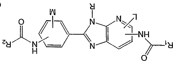
Genus D1;
