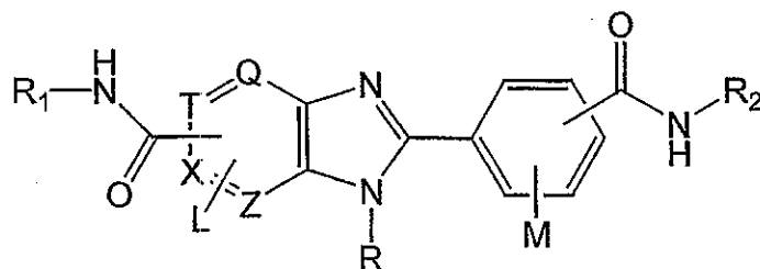
Supragenus B;
