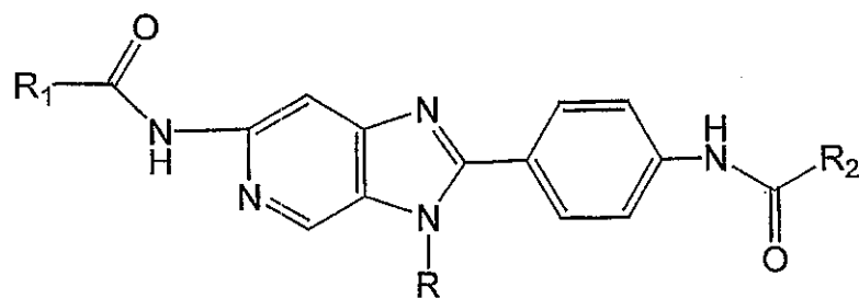
Subgenus D2a;
