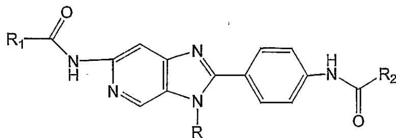
Subgenus D2a;
