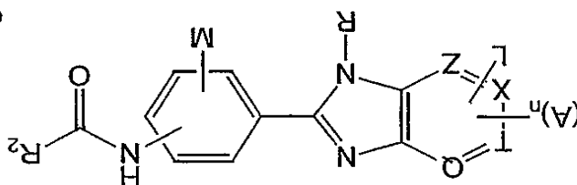
Genus A5
