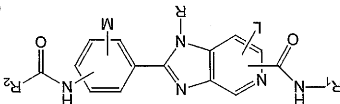
Genus A3
