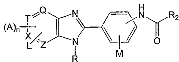
Genus A5
