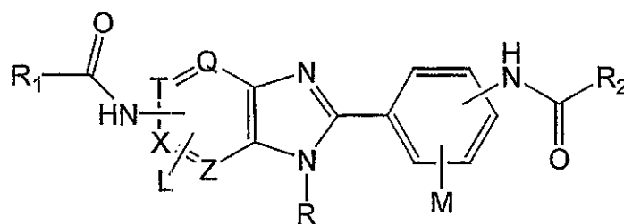
Supragenus D;
