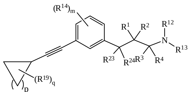
Formula (D)
