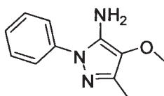
4-methoxy-3-methyl-1-phenyl-1H-pyrazol-5-amine
