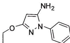
3-ethoxy-1-phenyl-1H-pyrazol-5-amine
