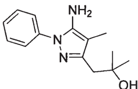
1-(5-amino-4-methyl-1-phenyl-1H-pyrazol-3-yl)-2-methylpropan-2-ol
