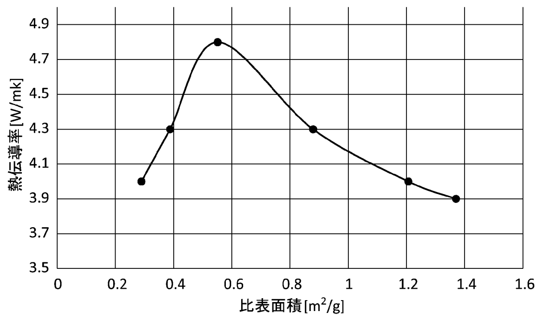
比表面積と熱伝導率の関係
