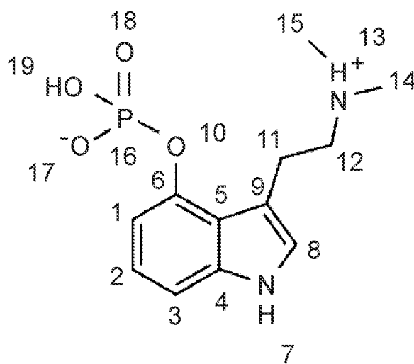
Psilocybin
