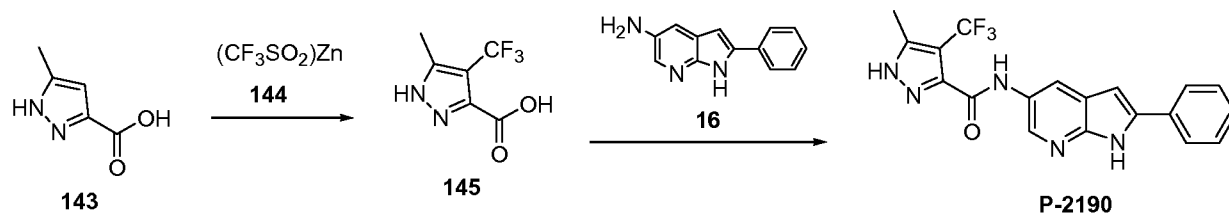
Scheme 25.
