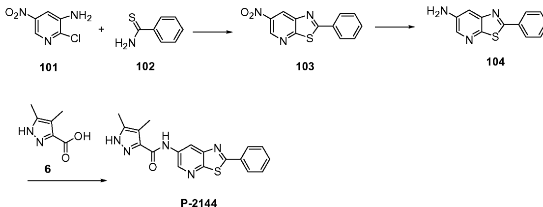
Scheme 17.
