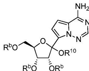
Formula (V-a),
