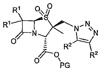
(IIa)
