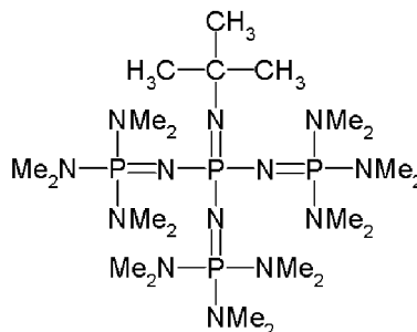
t-Bu-P4
