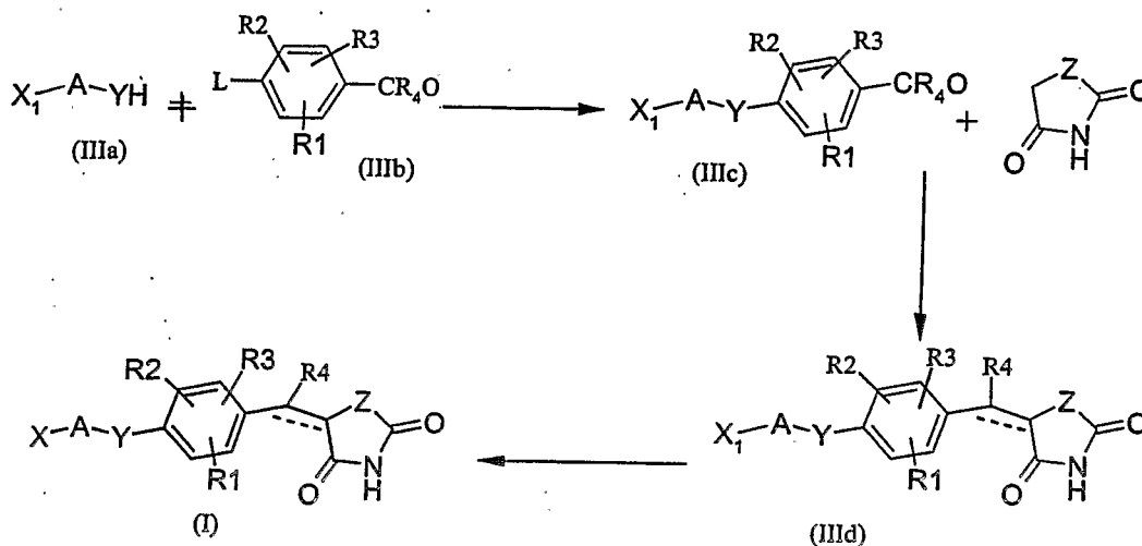
Scheme-I
