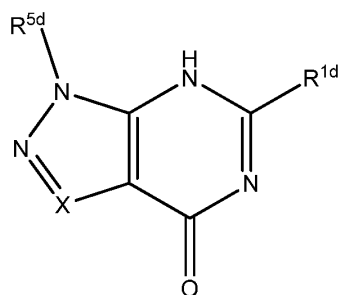
Formula VIId
