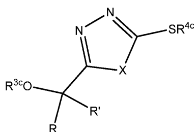
Formula Ic
