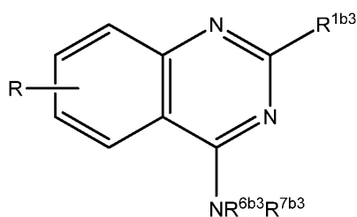
Formula VIIIb3
