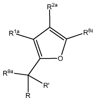
Formula Va
