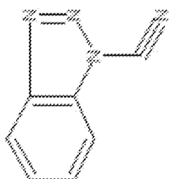
1-cyanobenzotriazole (1-CBT)
