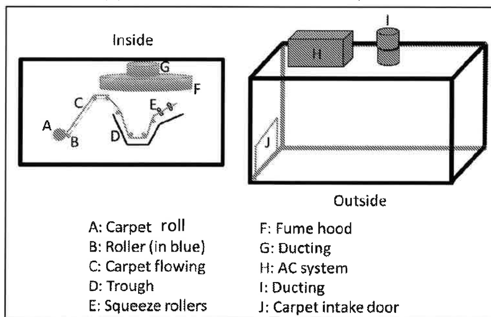
(d) Chamber for Solution Treatment System
