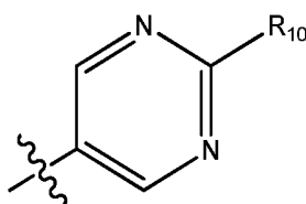
IIb
