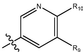
IIb
