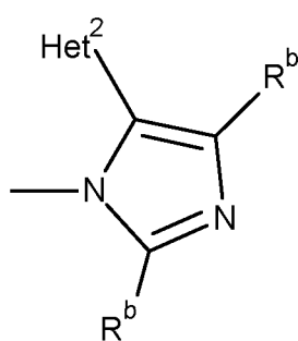
Het1/2l
