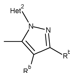
Het1/2m
