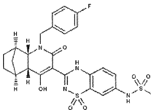
ANA-598 (Setrobuvir)
