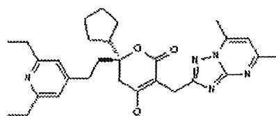
filibuvir (PF-00868554)
