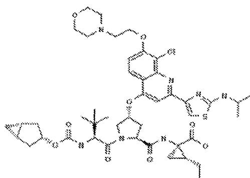
GS-9451
