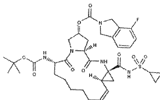
danoprevir
