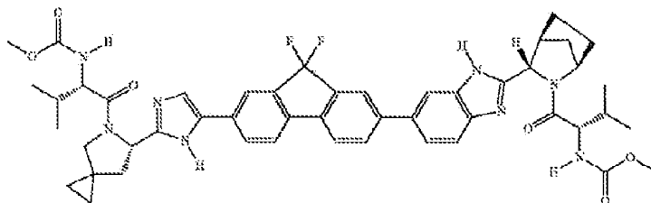
GS-5885
