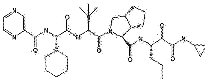
Telaprevir
