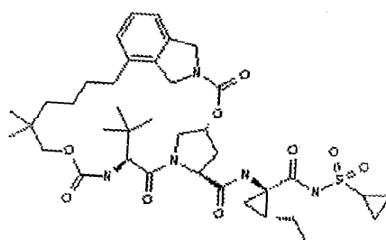
Vaniprevir, MK-7009
