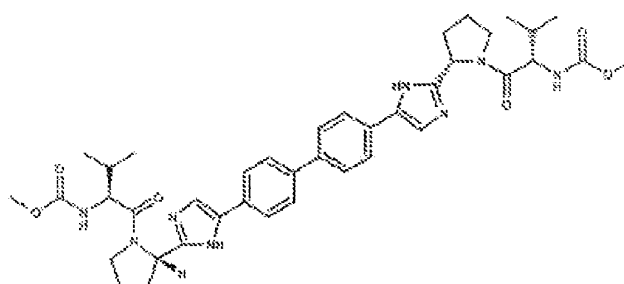
BMS-790052 (daclatasvir)
