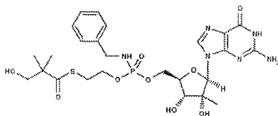
IDX-184
