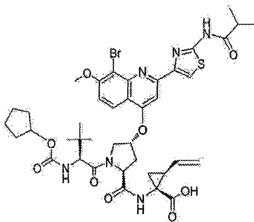
BI-201335
