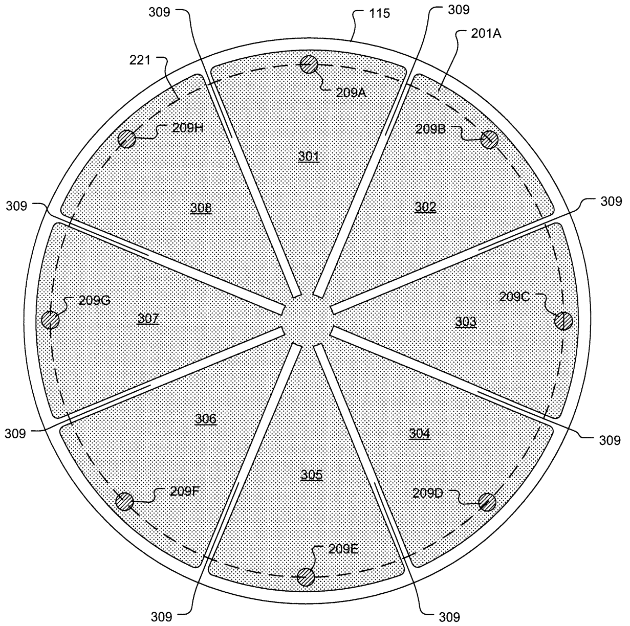
View A-A
