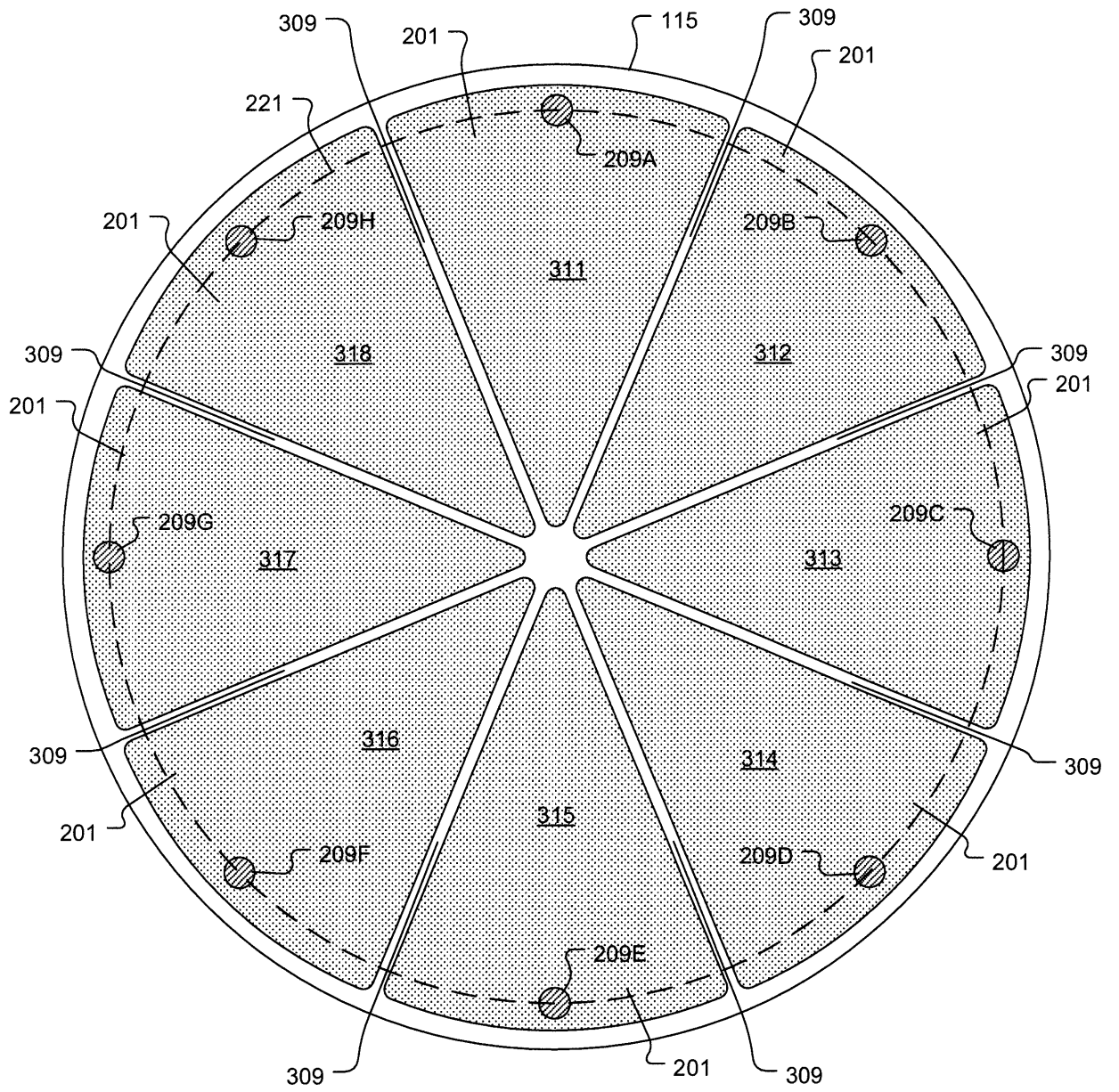
View A-A
