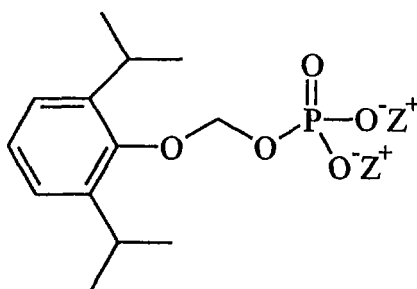
Propofol Prodrug
