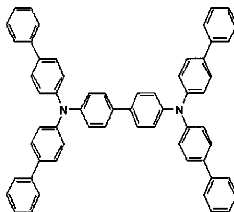
TBDB
