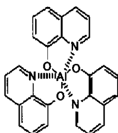
Alq
