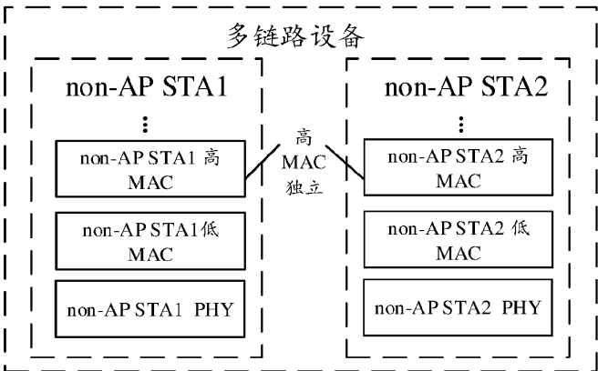
non-AP MLD: 非接入点多链路设备 non-AP STA: 非接入点站点 MAC: 媒体接入控制层 PHY: 物理层
