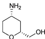
cis-(4-aminotetrahydro-2 H -pyran-2-yl)methanol
