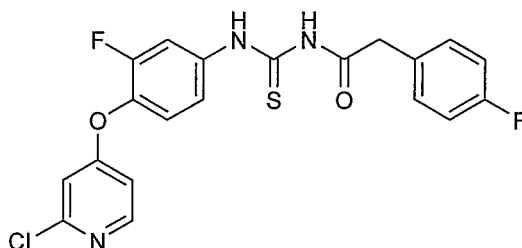
1-(4-(2-Chloropyridin-4-yloxy)-3-fluorophenyl)-3-(2-(4-fluorophenyl)acetyl)thiourea
