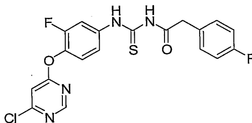
1-(4-(6-Chloropyrimidin-4-yloxy)-3-fluorophenyl)-3-(2-(4-fluorophenyl)acetyl)thiourea
