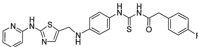
1-(2-(4-Fluorophenyl)acetyl)-3-(4-((2-(pyridin-2-ylamino)thiazol-5-yl)methylamino)phenyl)thiourea
