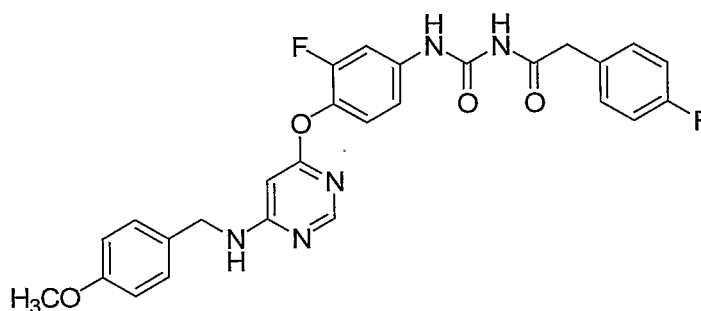
1-(4-(6-(4-Methoxybenzylamino)pyrimidin-4-yloxy)-3-fluorophenyl)-3-(2-(4-fluorophenyl)acetyl)urea
