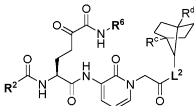
(IV-g)
