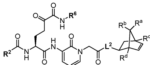
(IV-h)
