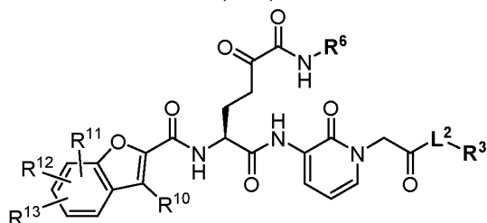
(V-d)
