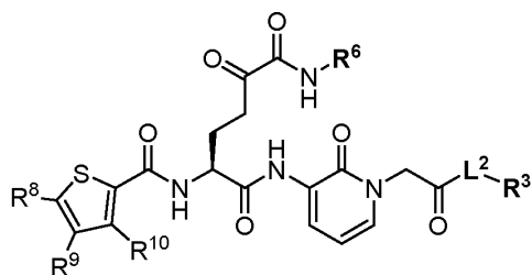
(V-b)
