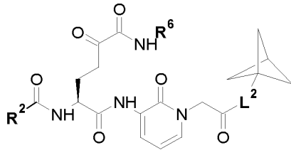
(IV-m)
