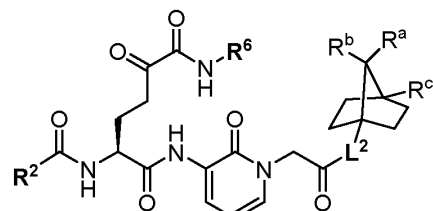
(IV-f)
