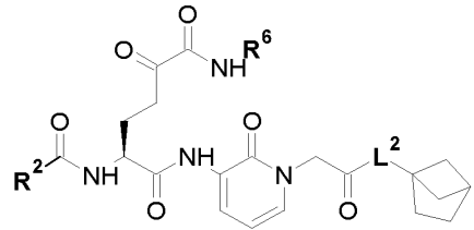
(IV-n)
