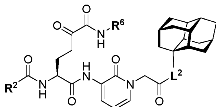
(IV-k)
