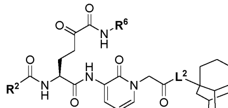
(IV-j)
