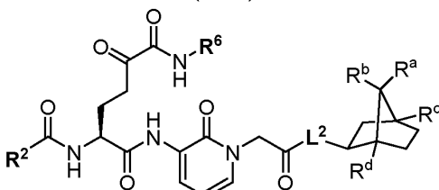
(IV-e)
