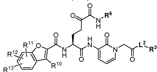
(V-d)
