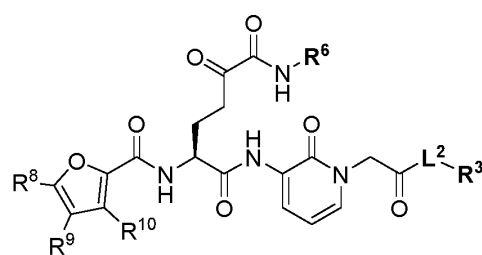
(V-a)
