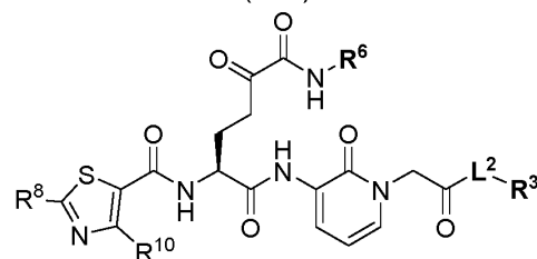
(V-c)
