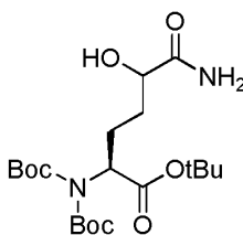
(2S)-tert-butyl 6-amino-2-(bis(tert-butoxycarbonyl)amino)-5-hydroxy-6-oxohexanoate
