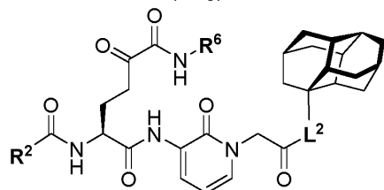
(IV-l)
