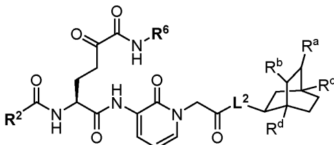
(IV-i)
