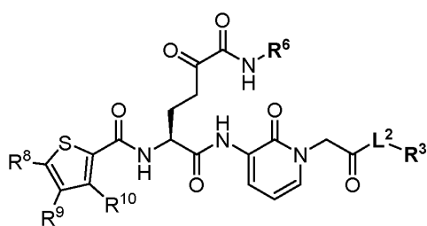
(V-b)
