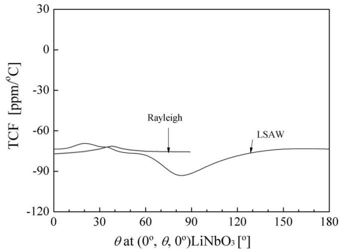
FIG. 20(c) (0^\circ, \theta, 0^\circ) LN
