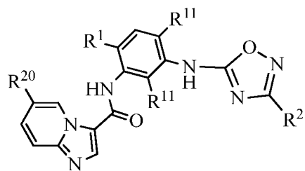
Formula (Ile)
