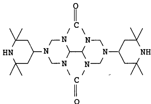
Uvinul® 4049 H
