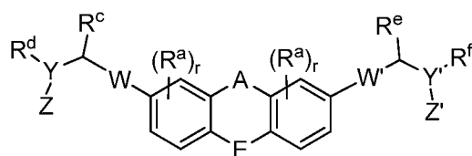
IIa.
