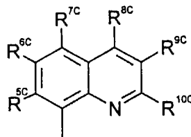
8-quinolyl
