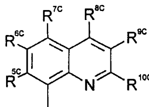
8-quinolyl
