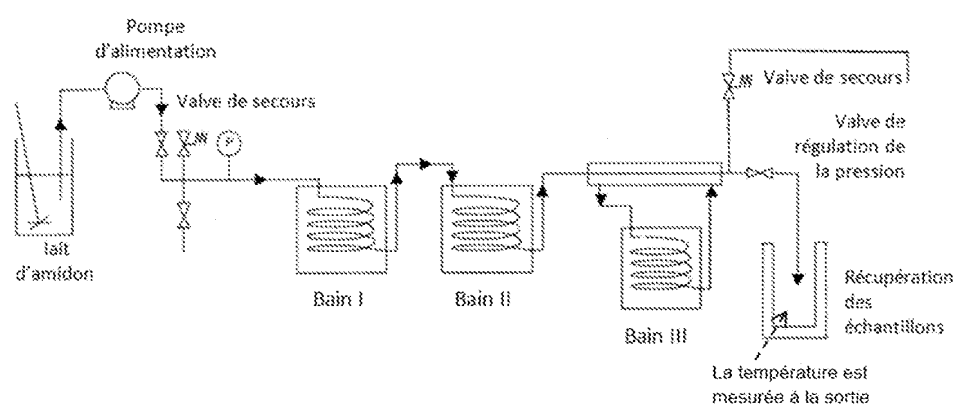
Le Réacteur Continu
