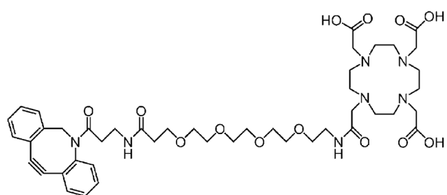
DO3A-PEG4-DBCO
