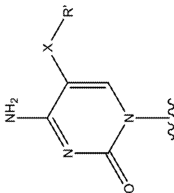
CYTOSINE
