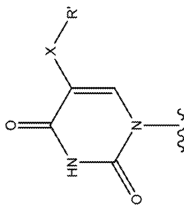
URACIL
